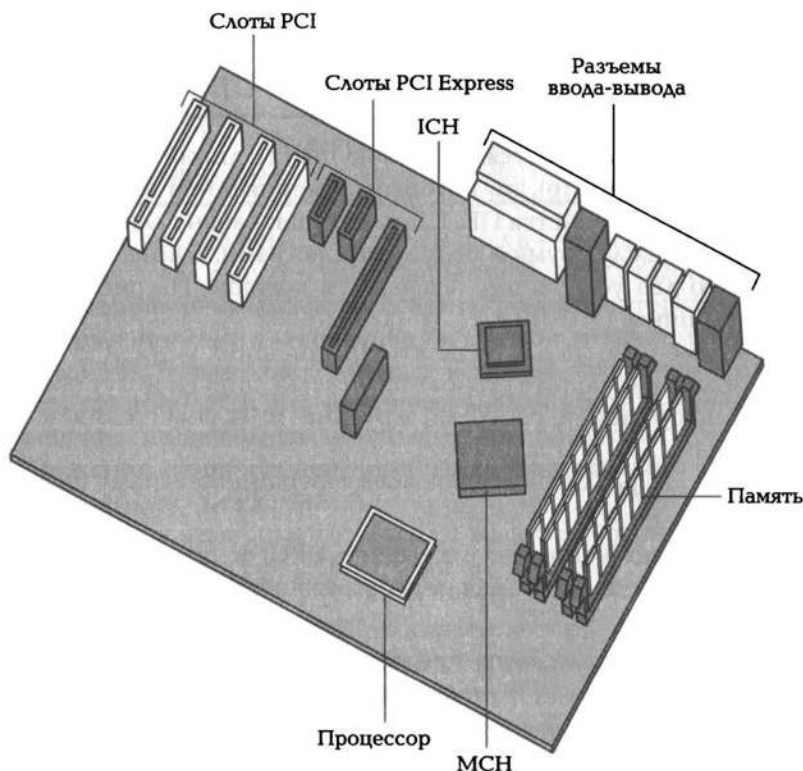
Рис. 2.6. Расположение элементов на системной плате в соответствии со спецификацией ATX
