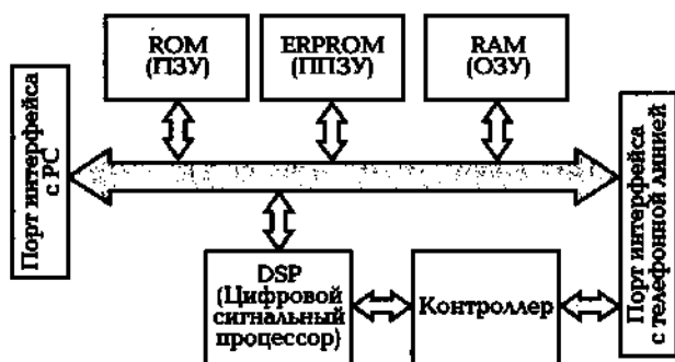
Рис. В.10. Структурная схема модема
