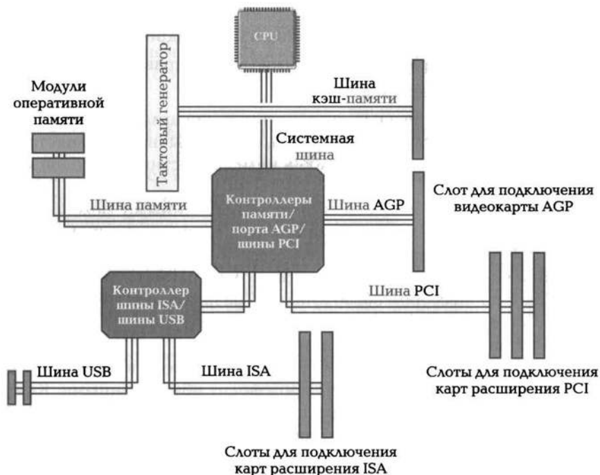
Рис. 2.7. Структура шины
