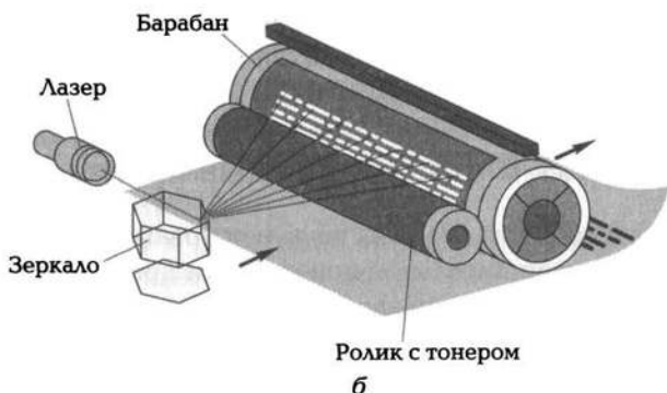
Рис. 7.4. Лазерный принтер:
