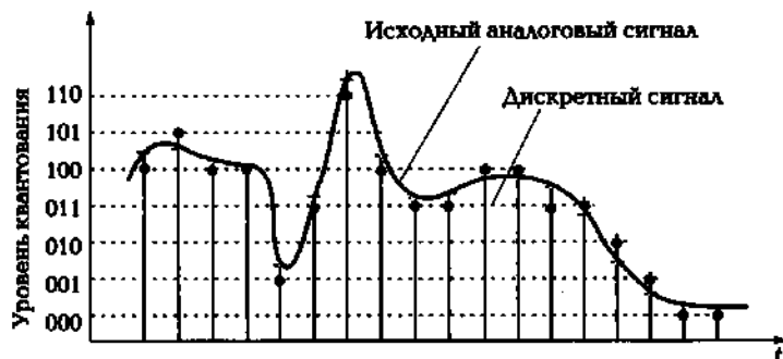
Рис. 5.3. Дискретизация по времени и квантование по уровню аналогового сигнала
