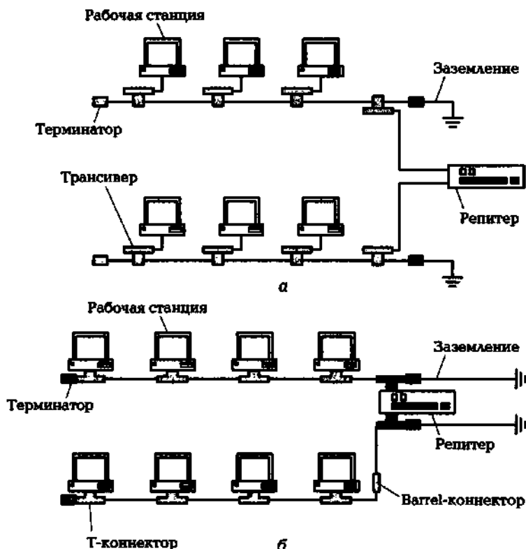
Рис. 8.6. Сеть Ethernet:
