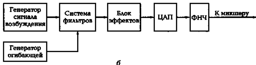
Рис. 5.5. Принцип действия современного синтезатора:
