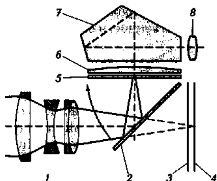
Рис. 6.13. Схема зеркального цифрового фотоаппарата:
