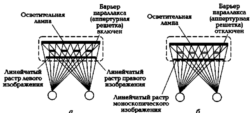
Рис. 4.18. Схема принципа действия апертурно-растрового автостереодисплея:
