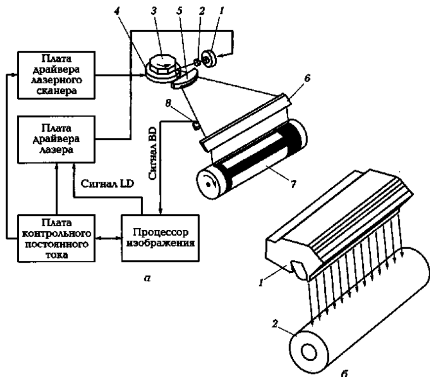
Рис. 9.3. Схемы записи изображения в цифровых электрографических копируемых аппаратах:
