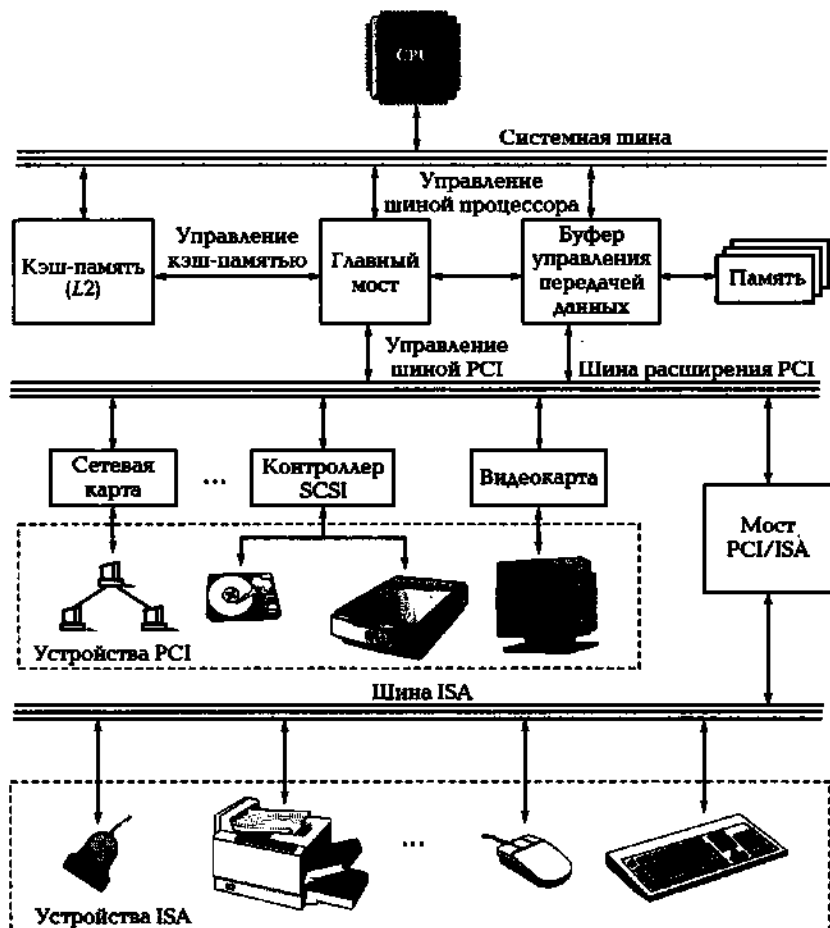
Рис. 2.В. Архитектура шины PCI
