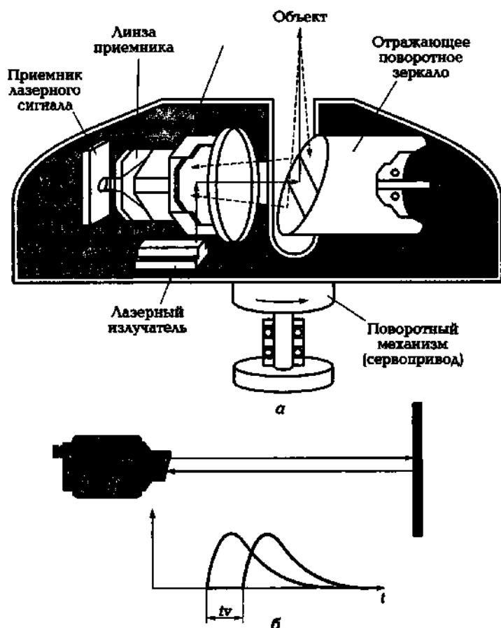
Рис. 6.10. Лазерный 3D-сканер:
