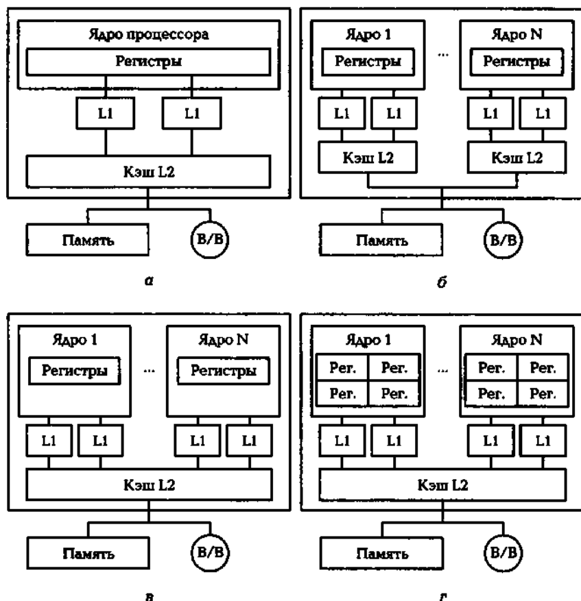
Рис. 2.13. Варианты архитектур CMP:
